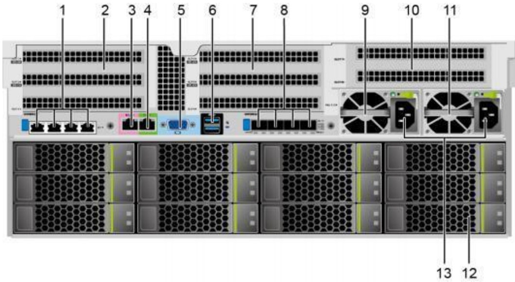
图 4.2：后面板组件
