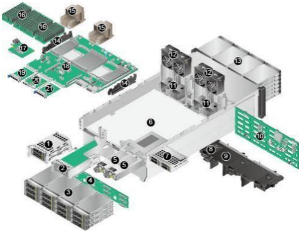
图4. 17：物理结构（配置鲲鹏 920 7260、5250处理器）
