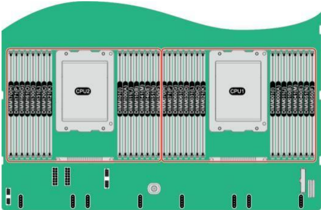
图 6.1：DIMM 安装位置（鲲鹏 920 7260、5250处理器）
