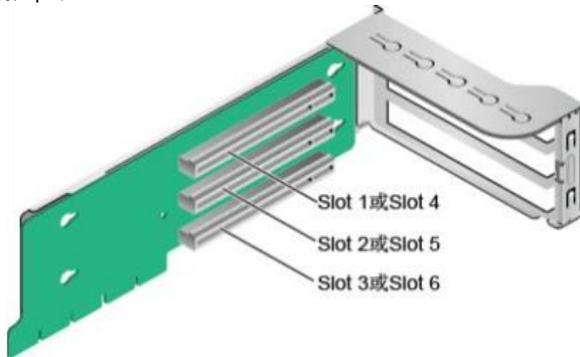
图 4.9: 3x8 Riser 卡 1
