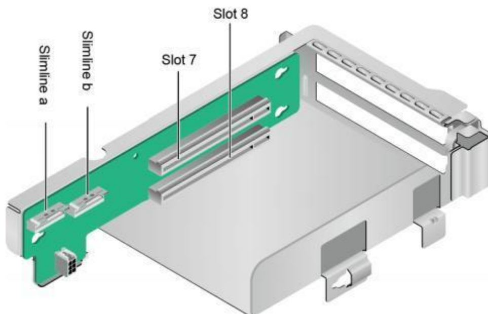
图 4.12 2x8 Riser 卡 6（板名：BC82PRUF）
