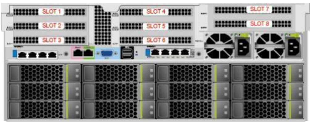
图 4.14：PCIe 插槽
