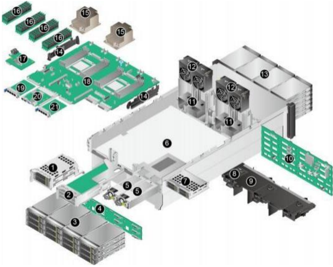
图 4.18：物理结构（配置鲲鹏 920 5220 或 3210 处理器）
