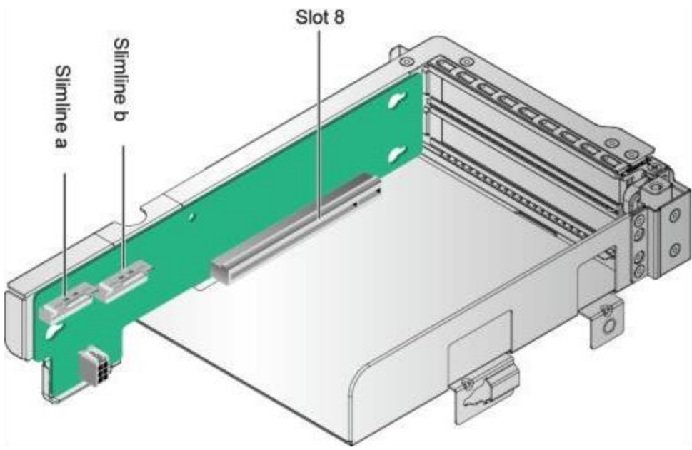
图 4.13：1x16 Riser 卡 7
