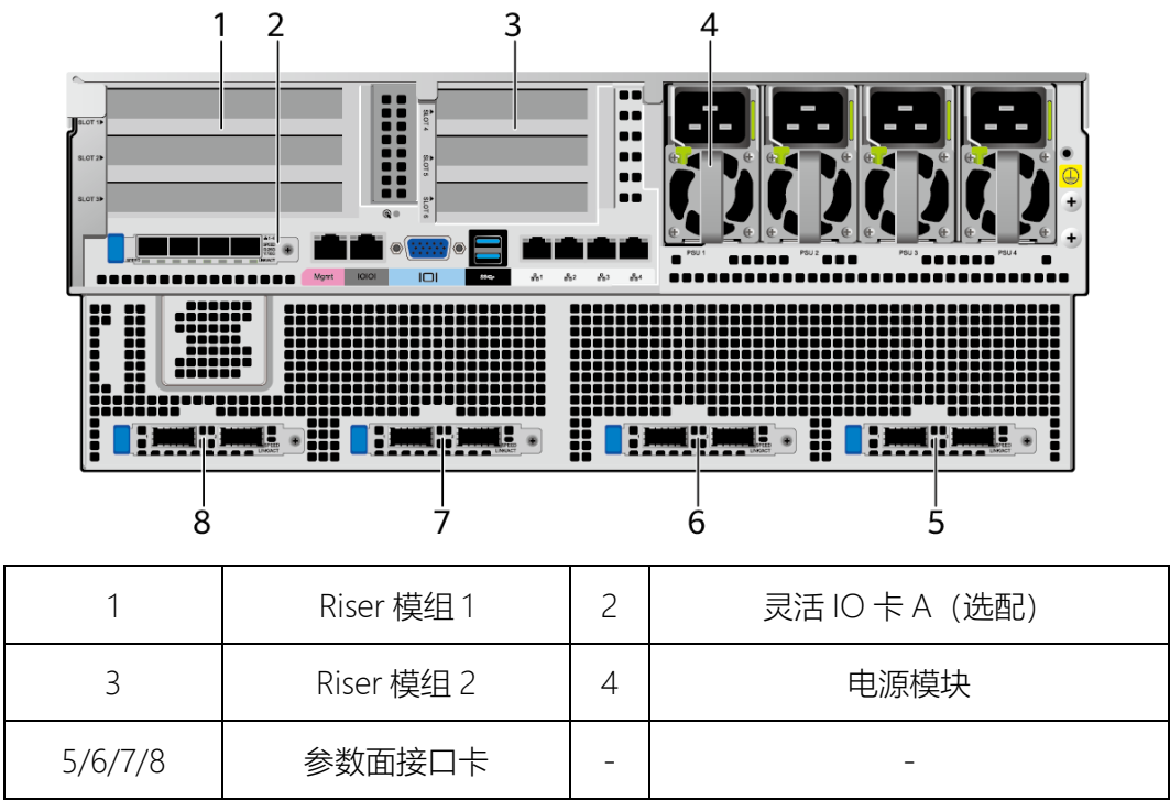
图4-3 后面板组件示意图
