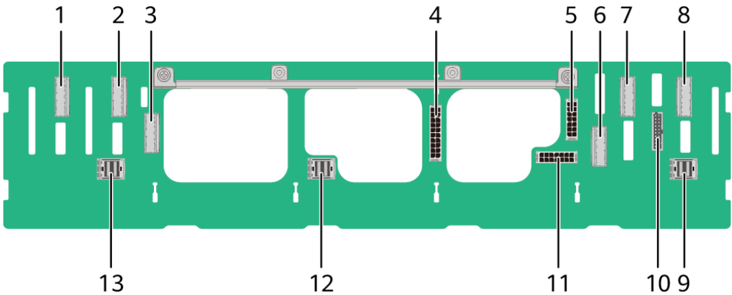
图4-15 硬盘背板
