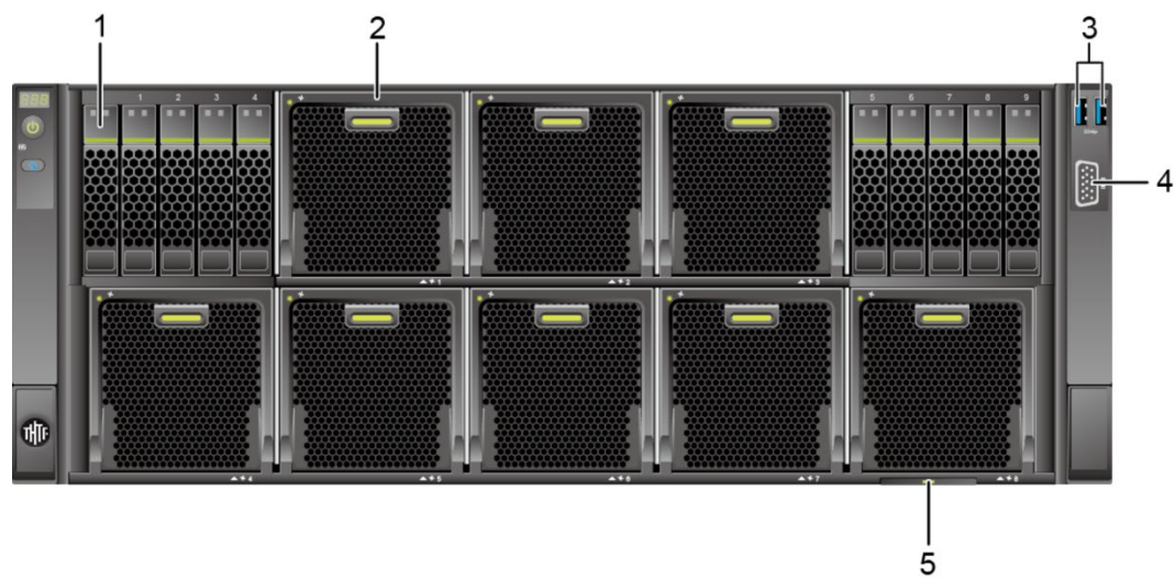
图4-1 前面板组件示意图
