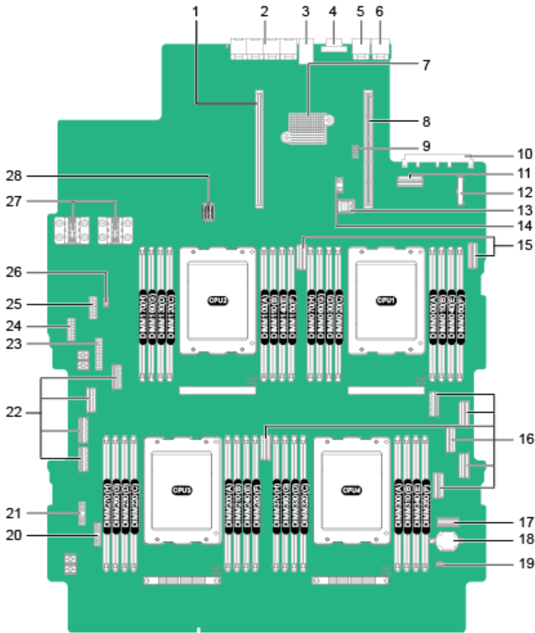
图4-16 主板接口
