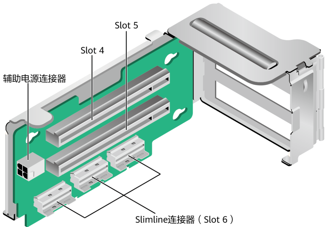
图4-12 Riser 卡 2 示意图
