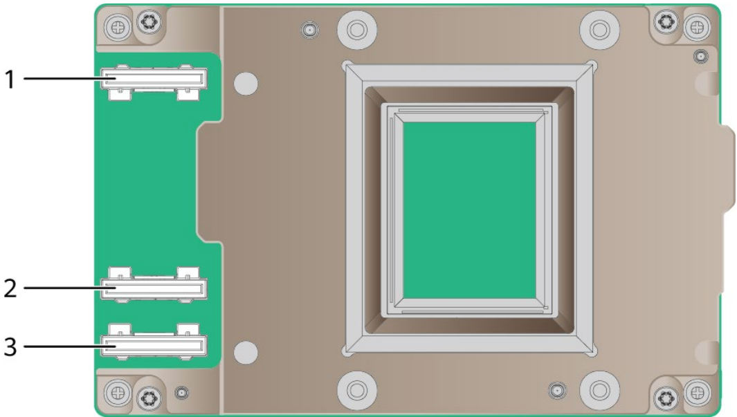
图4-17 NPU 模组接口示意图
