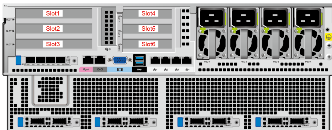
图4-10 PCIe 插槽位置
