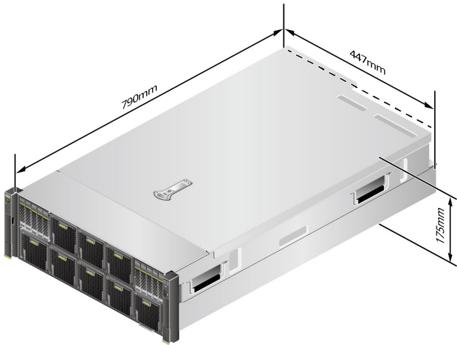
图5-1 物理尺寸示意图
