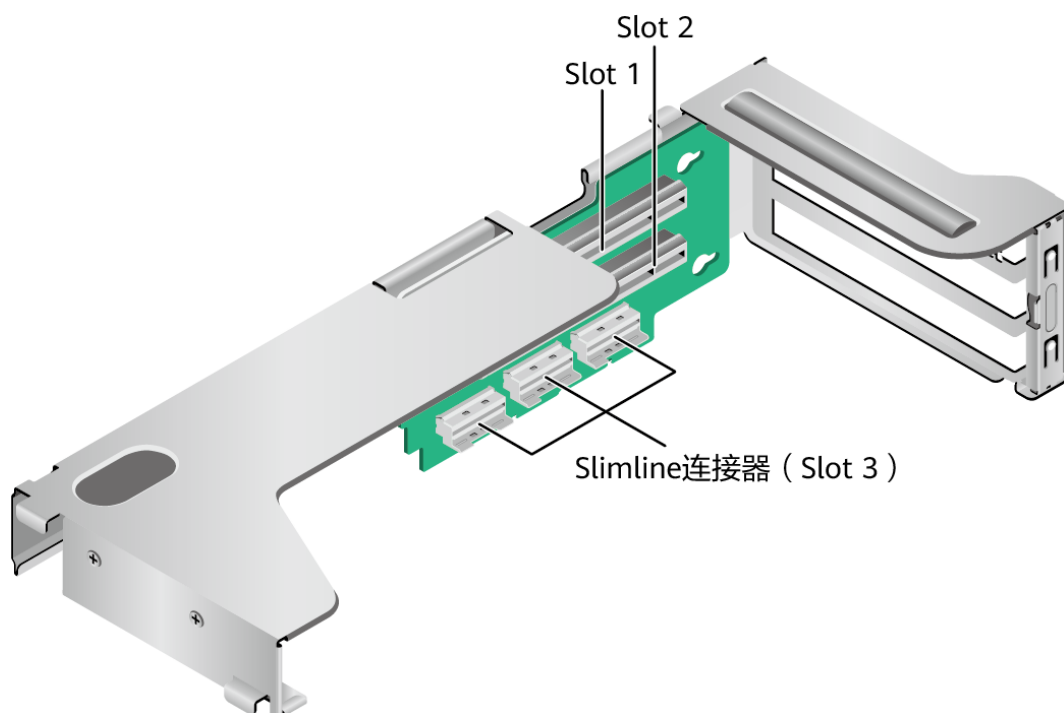
图4-11 Riser 卡1示意图
