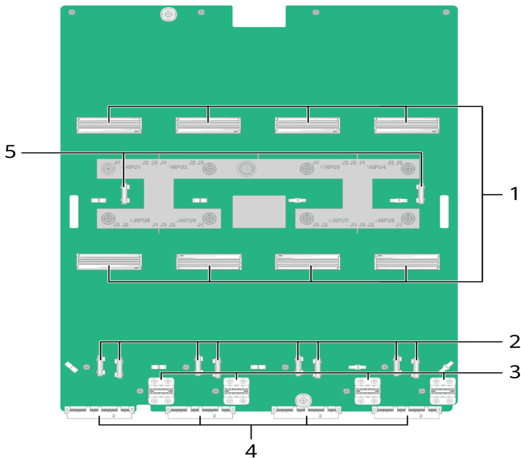
图4-18 NPU 板接口
