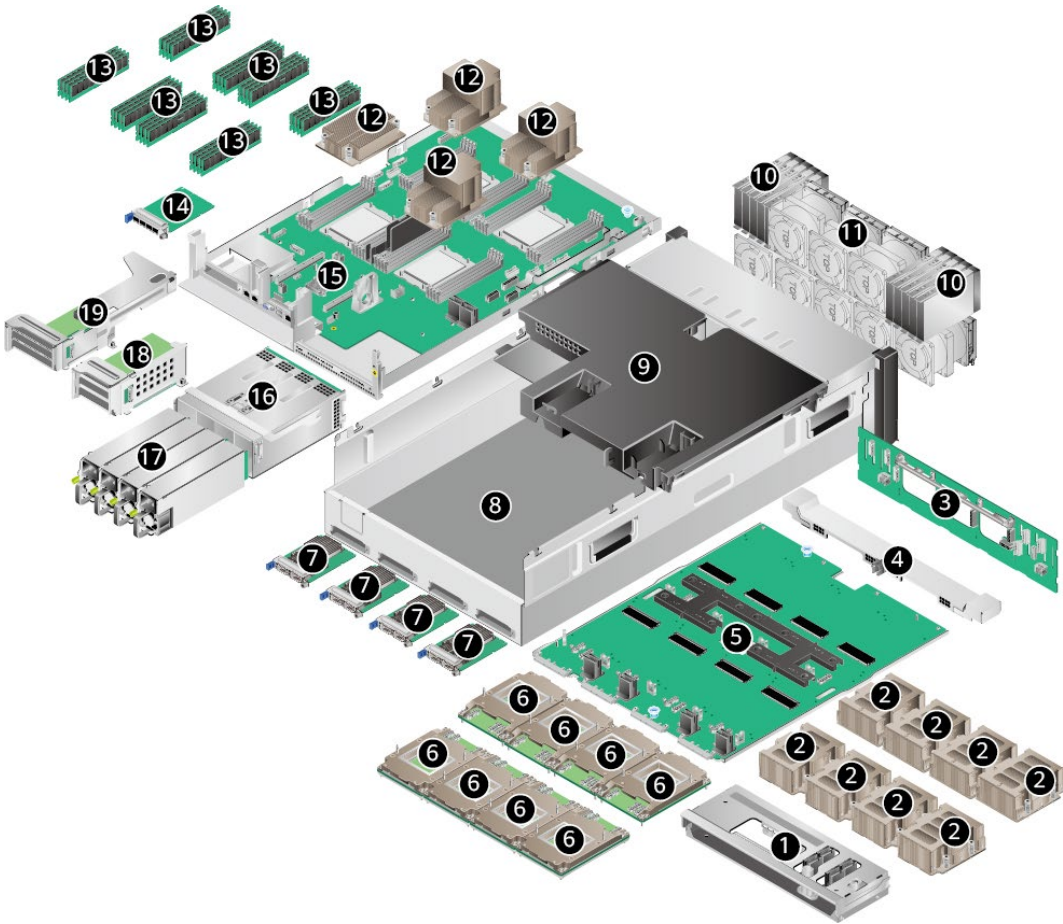
图3-1 部件示意图
