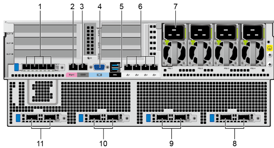
图4-4 后面板接口示意图
