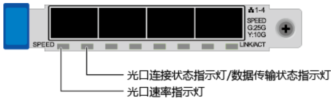
图4-13 TM280/TM281 (4*25GE/10GE 光口)
