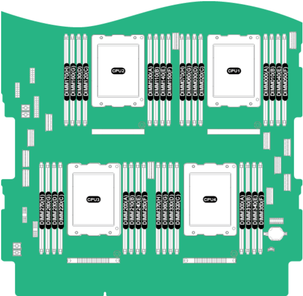
图 4-20 内存槽位编号
