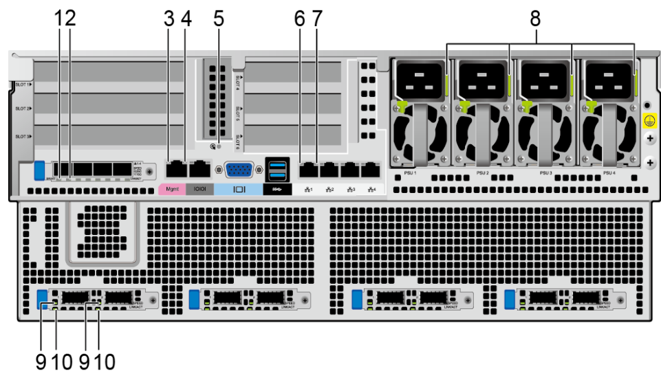
图4-5 后面板指示灯示意图
